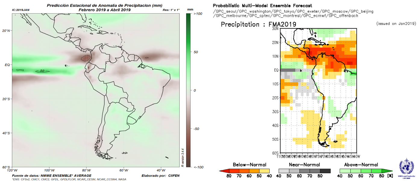
Fig.11 Izquierda: Pronóstico estacional de lluvias (anomalías en mm) Febrero – Abril 2019. Fuente de datos: NMME/CPC/NOAA. Procesamiento: CIIFEN Derecha: Pronóstico probabilístico Multi-Model Ensemble de lluvias Febrero – Abril 2019. Fuente: WMO Lead Centre - LRFMME.
