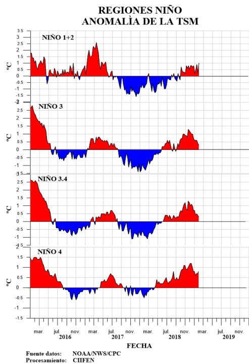
Fig. 3 Izquierda: Anomalía de la TSM en las Regiones NIÑO. Centro: Valor de la anomalía de la TSM en las regiones NIÑO y su cambio entre la semana de enero 02 de 2019 y enero 30 de 2019. Derecha: Ubicación de las regiones NIÑO en el Pacífico Ecuatorial.
