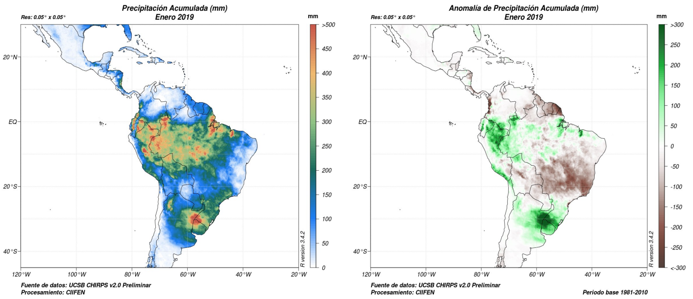
Fig. 8 Panel izquierda.- Precipitación mensual (mm). Panel derecha.- Anomalías de precipitación enero 2019 (mm) Fuente: UCSB CHIRPS v2.0 Preliminar
