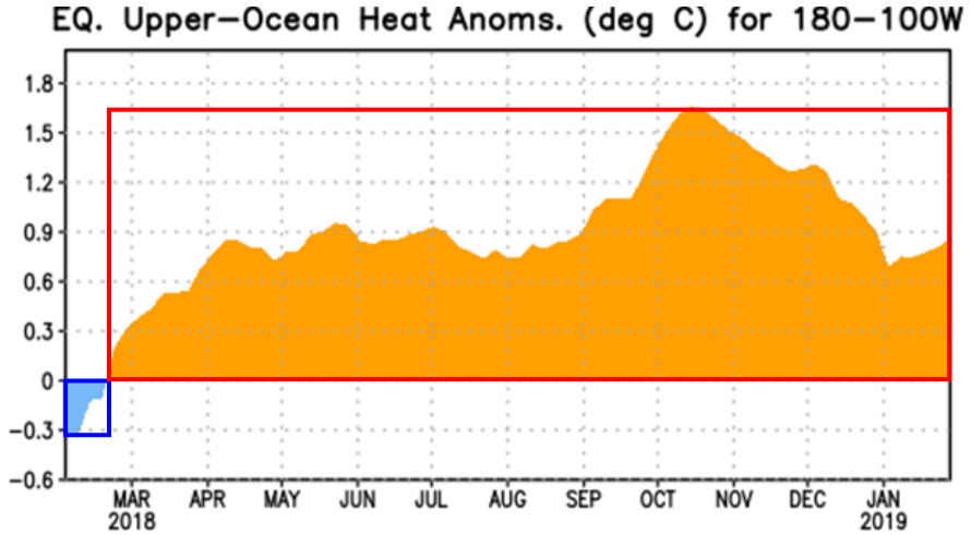
Fig. 4 Anomalía de Calor (°C) en la capa superior (0 a 300 m) del Pacífico ecuatorial central-Oriental (entre 180° -100°W). Fuente de información: CPC/NCEP
